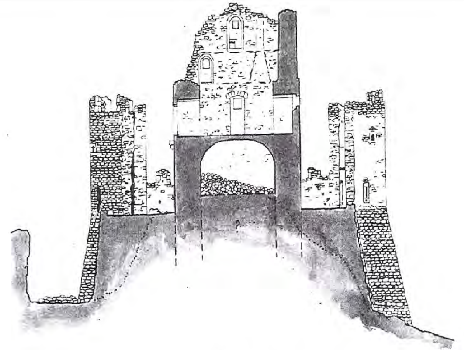
SEZIONE A-A
